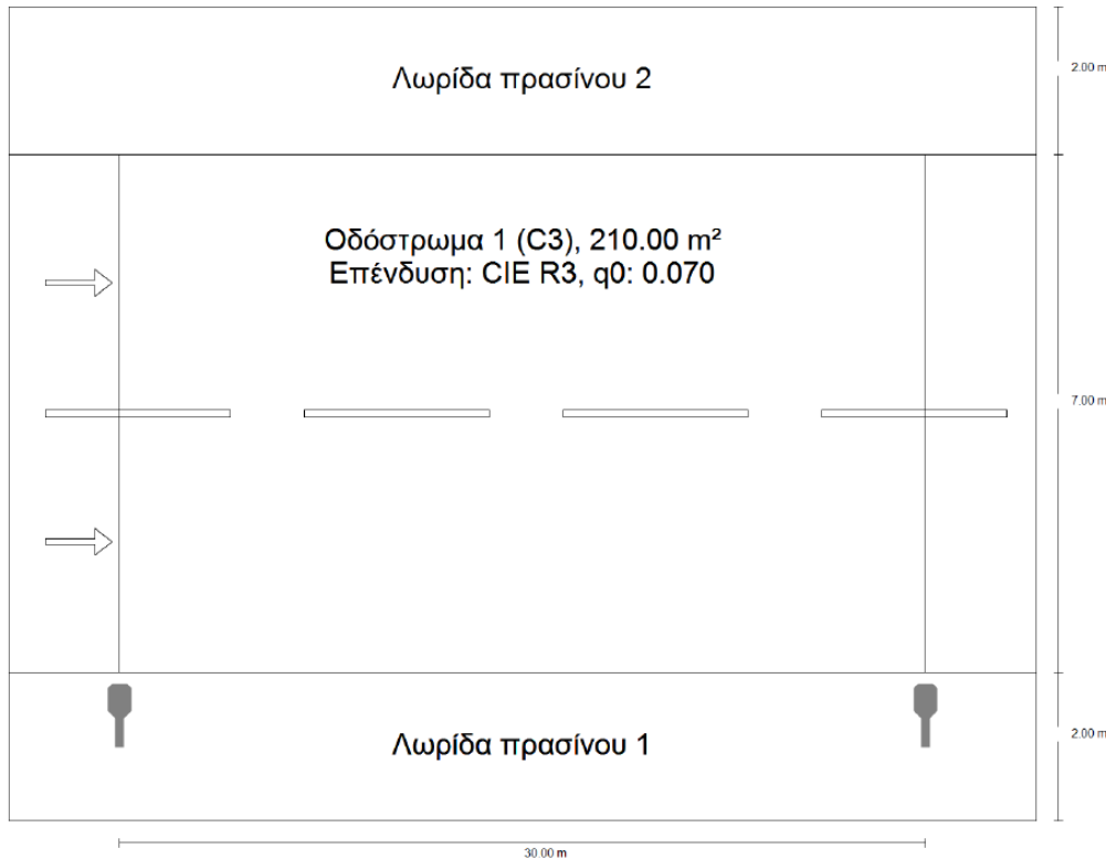
Εικόνα 2 Διάταξη φωτοτεχνίας
